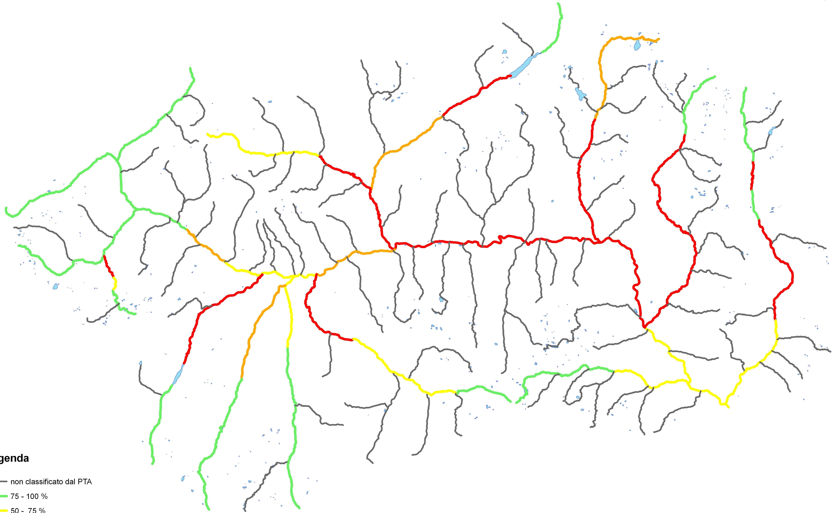
Fig. 2.4 Quantità residua %di acqua in riferimento al bilancio idrico del PTA
