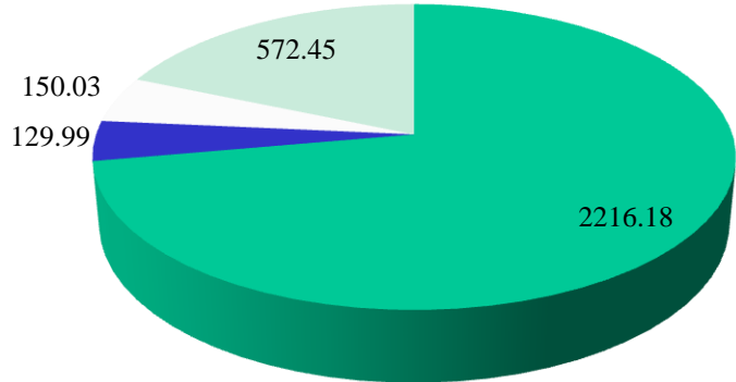
CO (t/anno)
