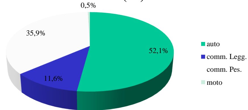
NOx (%)
