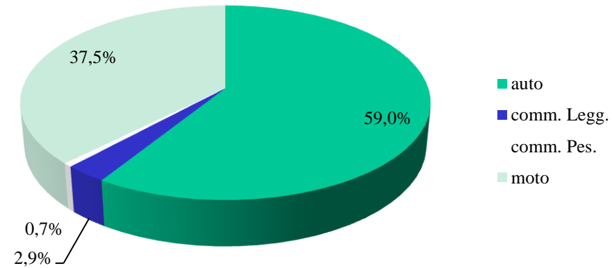
benzene (%)
