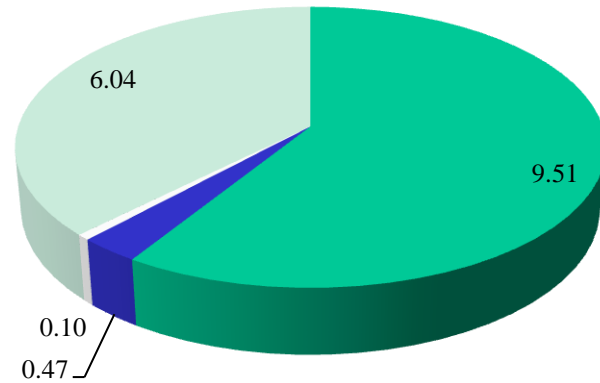
benzene (t/anno)
