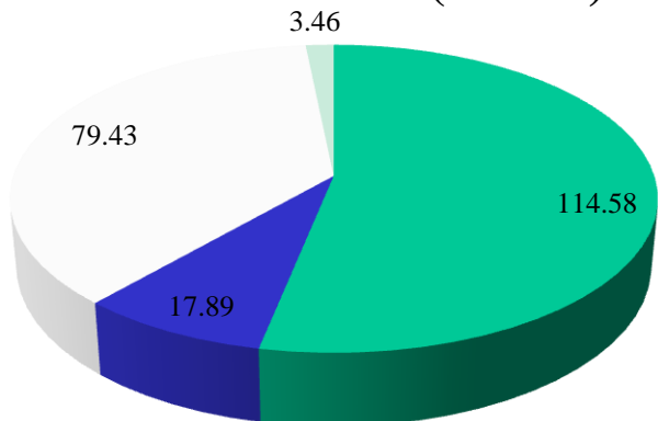
PM10 (t/anno)
