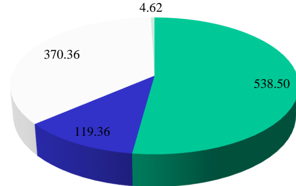
NOx (t/anno)
