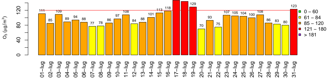
Donnas – O 3 massimo della media mobile su 8 ore
