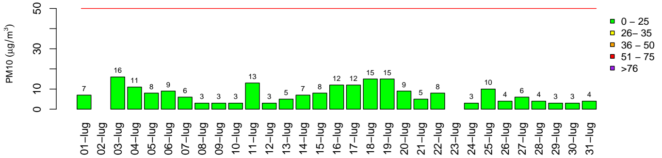
Donnas – PM10 Media giornaliera
