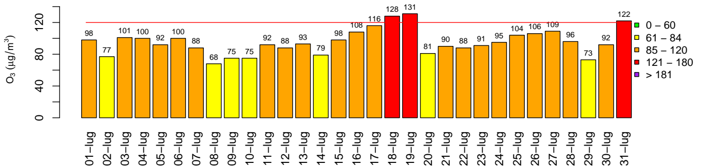
Aosta – Mont Fleury – O 3 massimo della media mobile su 8 ore
