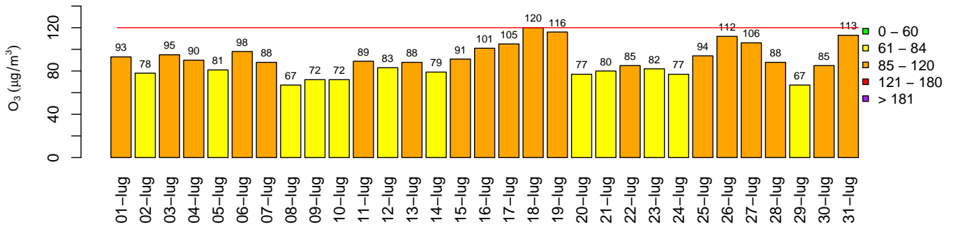
Aosta – Piazza Plouves – O 3 massimo della media mobile su 8 ore
