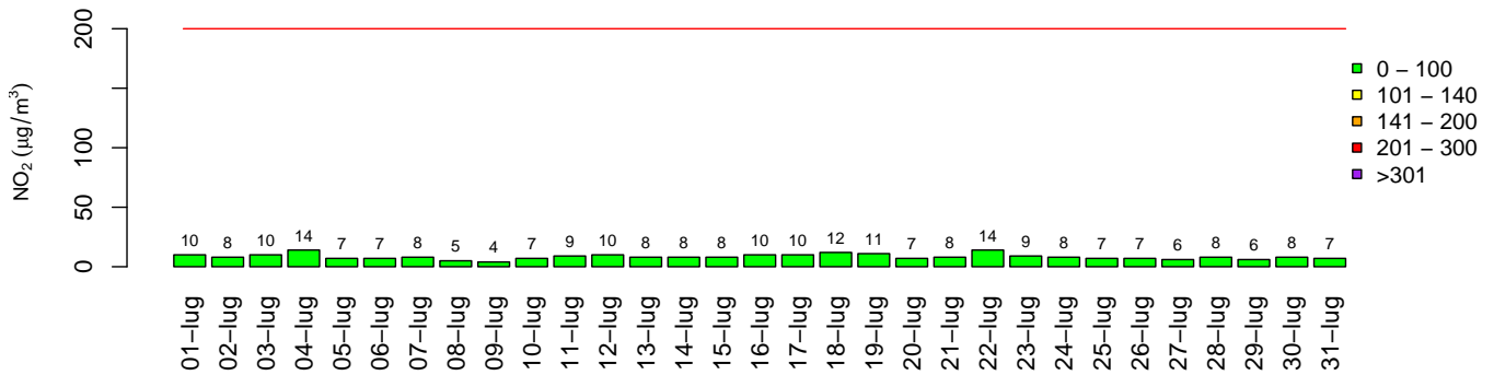
Donnas – NO 2 Massimo Media oraria
