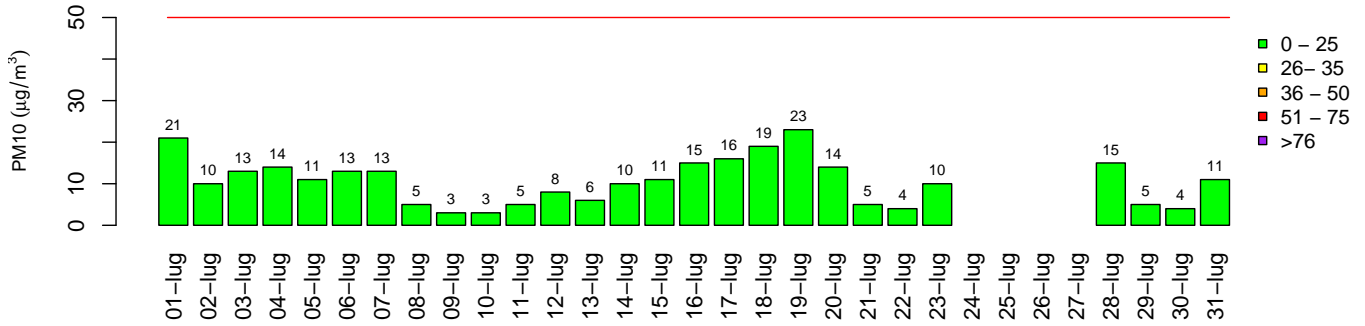
Aosta – Piazza Plouves – PM10 Media giornaliera
