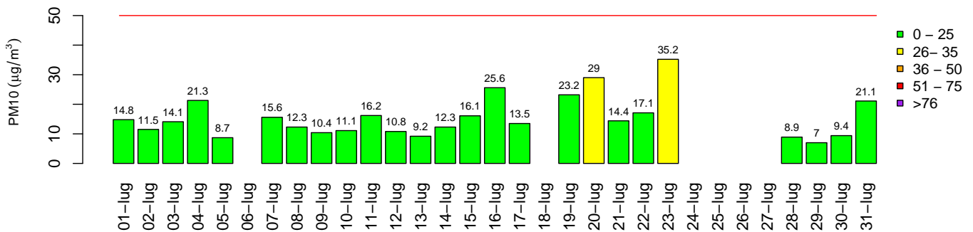
Aosta – Pepinière – PM10 Media giornaliera
