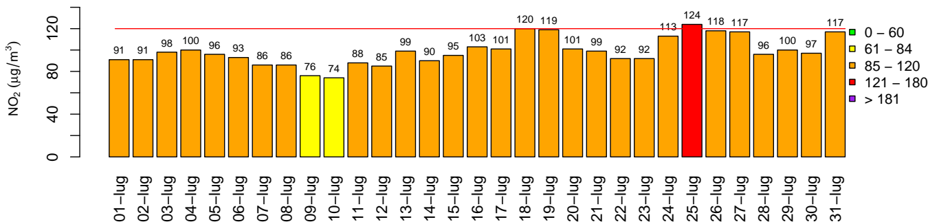
La Thuile – O 3 massimo della media mobile su 8 ore
