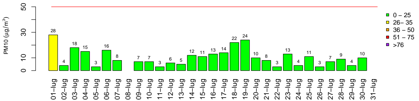
Aosta – Quartiere Dora – PM10 Media giornaliera
